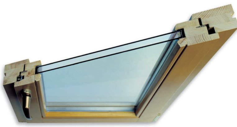
Řez oknem EURO
