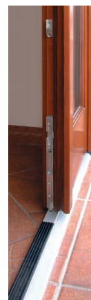
Detail Al prahu a zástrčky dvoukřídlých dveří EURO
